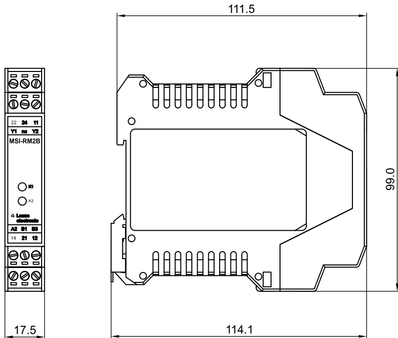
Рис. 13.1: Размеры MSI-RM2B-01
