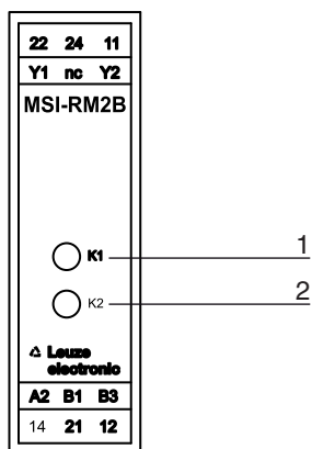
Рис. 3.4: Индикаторы MSI-RM2B
